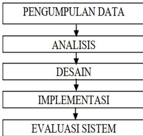
Gambar 1. Tahap Penelitian
